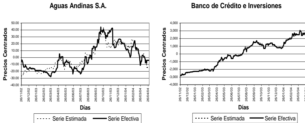
Figura 4 - Comparación de la Serie Original con la Aproximación con Cinco Factores.
