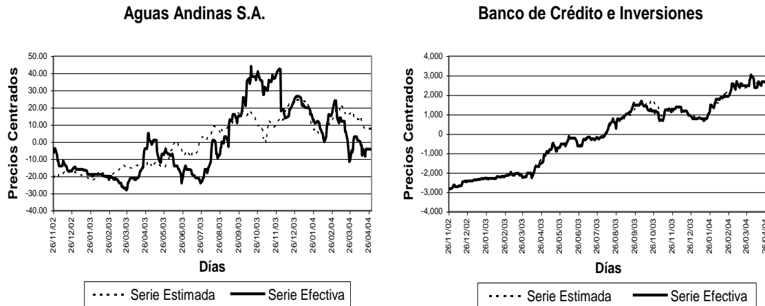
Figura 3 - Comparación de la Serie Original con la Aproximación con Tres Factores.
