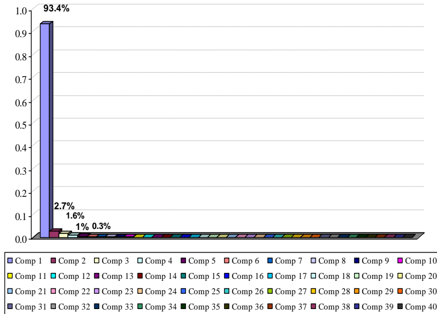
Figura 2: Importancia Relativa de los Factores
